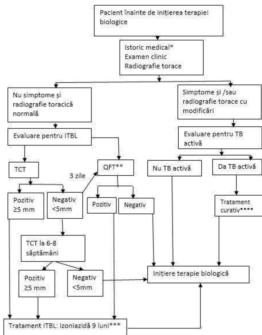
Algoritm de diagnostic ITBL la copiii supuși terapiei biologice
